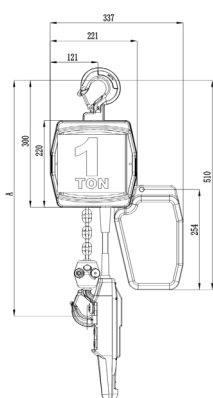
YJL 吊钩式, 250-2000kg
