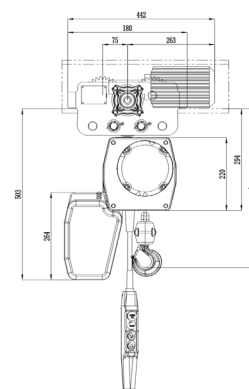
YJL 电动小车式 (十字型), 250-2000kg
