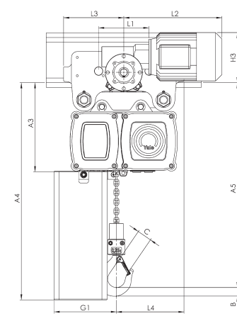
CPVF 集成式电动小车
