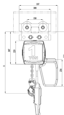
YJL 手推小车式 (十字型), 250-2000kg
