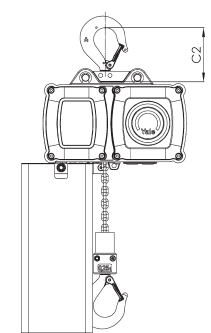
CPVF 悬挂吊钩式, 125 - 2500 kg
