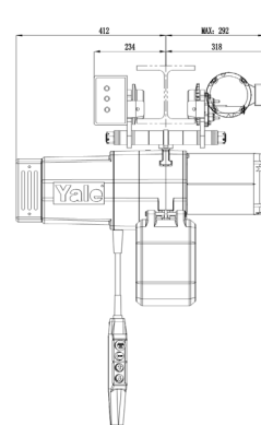
YJL 电动小车式 (十字型), 250-2000kg
